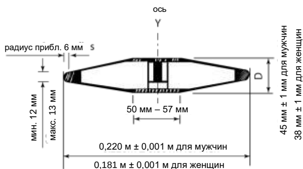
Рисунок ТП34 – диск
