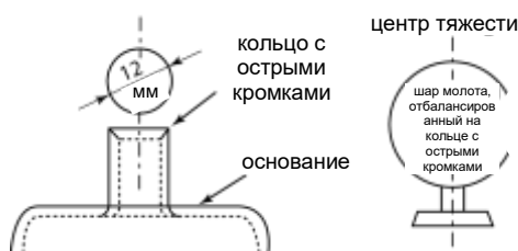
Рисунок (а) правило ТП36 – вариант устройства для проверки центра тяжести шара молота
